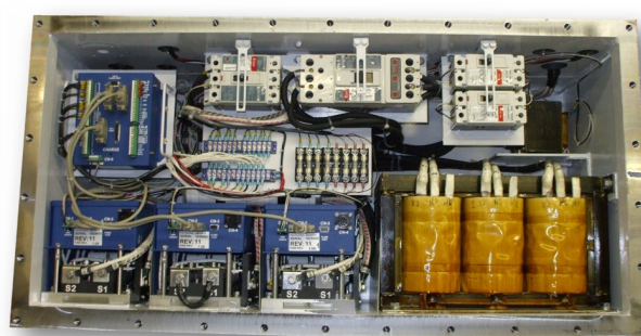
穿梭式机动矿车 三驱动器系统
