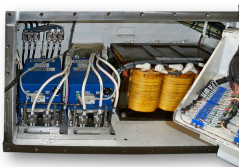
连续采煤机 双驱动器系统
