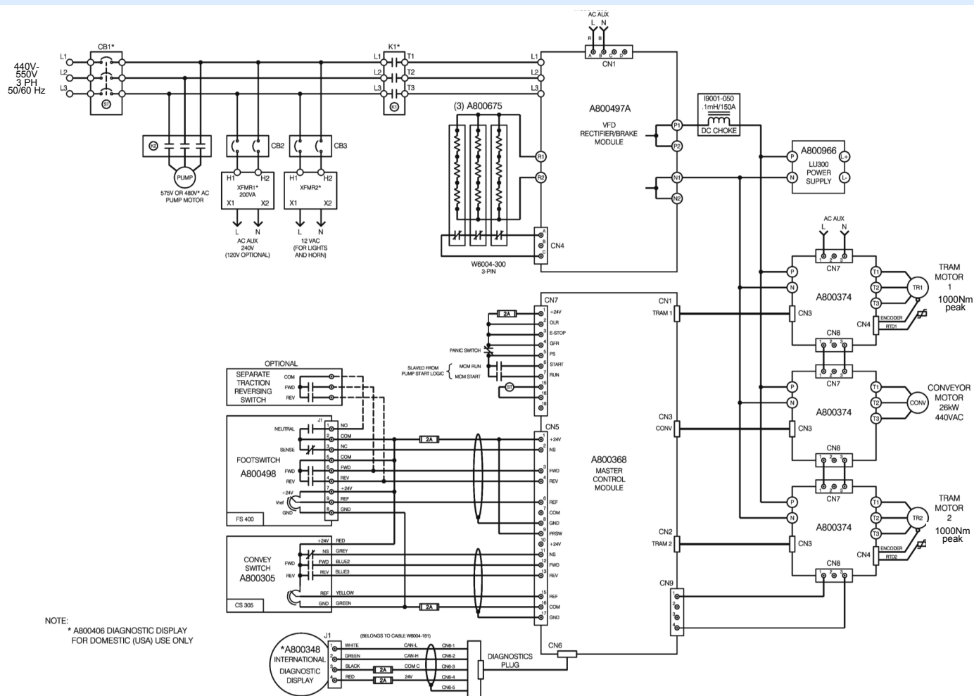
440V / 550V AC/AC 变频系统样本结构图
